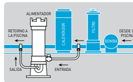
Ilustración del clorinador de tabletas modelo 300
