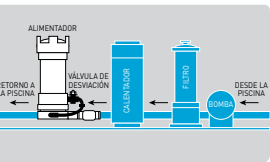
Ilustración del clorinador de tabletas modelo 320
