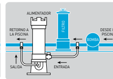
Ilustración del clorinador de tabletas modelo 300
